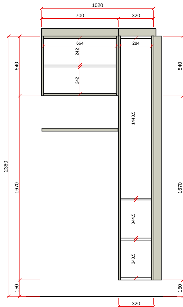
VISTA A - ESC. 1:20
