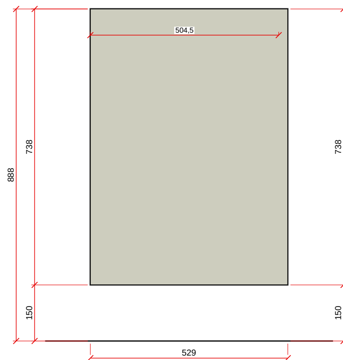
VISTA B - ESC. 1:10
